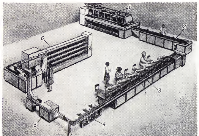
Рис. 1. Автоматизированная линия обработки письменной корреспонденции (ФРГ): 1 — машина для разборки писем по габаритам; 2 — лицовочно-штемпелевальная машина; 3 — аппараты для кодирования адресов писем — преобразования цифр и букв кода в условные люминесцентные знаки (точки или чёрточки); 4 — промежуточные накопители писем; 5 — читающее устройство пишмосортировочной машины; 6 — автоматическая пишмосортировочная машина.
